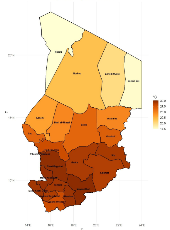
Température Moyenne - Jan 2026
